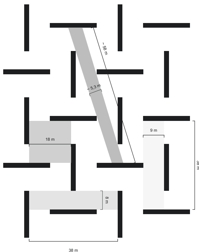
Figuur 7. Een hagelslagpatroon (variant 1, L=20\text{ m} , D=20\text{ m} , I=20\text{ m} , B=2\text{ m} en C=10\% ). De maximale ongedekte rechthoek is 18 \times 18\text{ m} ( =324\text{ m}^2 ). De maximale ongedekte ruimte in de lengterichting is 38 \times 9\text{ m} ( =342\text{ m}^2 ), loodrecht op de lengterichting 38 \times 8\text{ m} ( =304\text{ m}^2 ). In diagonale richting zijn er vier ongedekte ruimtes van circa 58 \times 5,3\text{ m} (ca. 307\text{ m}^2 ).
