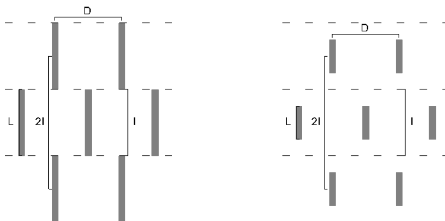
Figuur 2. De relatie tussen sleuflengte ( L ), sleufafstand ( D ) en sleufinterval ( I ). De stippellijnen geven de begrenzingen van de proefsleufrijen aan. Links een patroon met aansluitende proefsleufrijen, rechts een patroon waarbij de rijen niet aansluiten.
