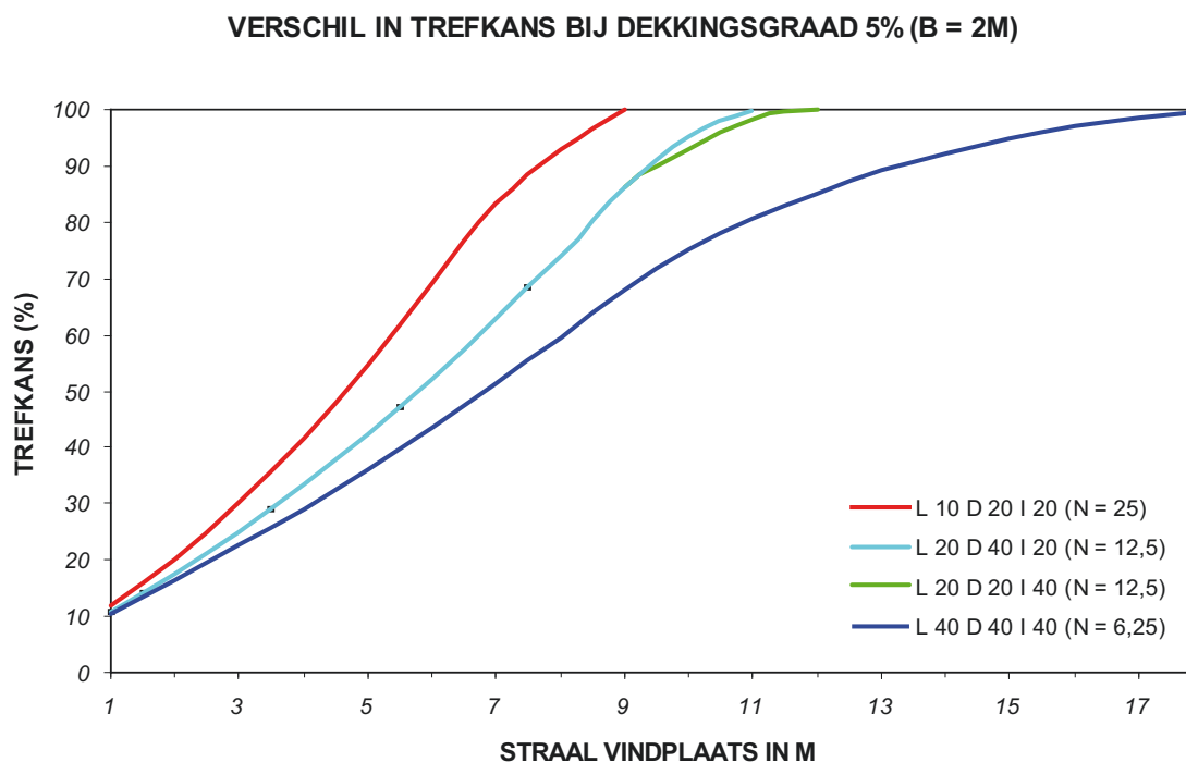
Figuur 4. Illustratie van de verschillen in trefkansen bij verschillende stippelijnpatronen met gelijke dekkingsgraad. B = sleufbreedte, L = sleuflengte, D = sleufafstand, I = interval, N = aantal sleuven per hectare. Zie ook hierna.
